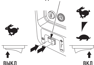
ВЫКЛЮЧАТЕЛЬ ЭКО-ДРОССЕЛЬНОЙ ЗАСЛОНКИ
